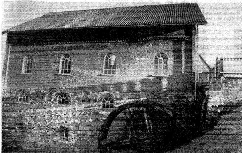
Extetal-Kükenbruch. Ein imposanter Anblick: die völlig restaurierte Mühle am Mühlenkamp. Das alte Mühlrad wurde mittlerweile demontiert und wird in Kürze durch das gleichgroße neue ersetzt. (Fotos [4]: Becker)
