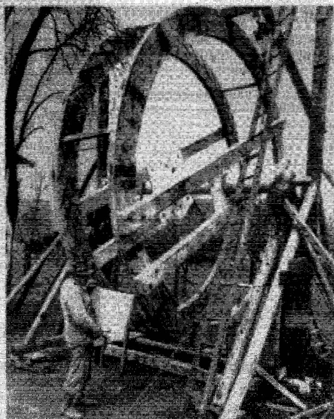
Kalletal-Bentorf/Harkemissen. Gustav Johanning hat viele Erfahrungen beim Mühlrad-Bau gesammelt. Das Foto zeigt ihn beim Einbau der „Schuffeln“ in das neue Rad, dessen Herstellung einige Monate dauert.
